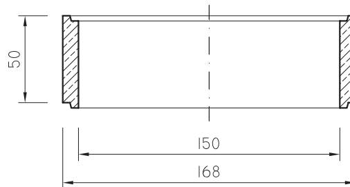
Schnitt
